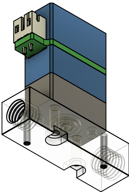
Silicone membrane
